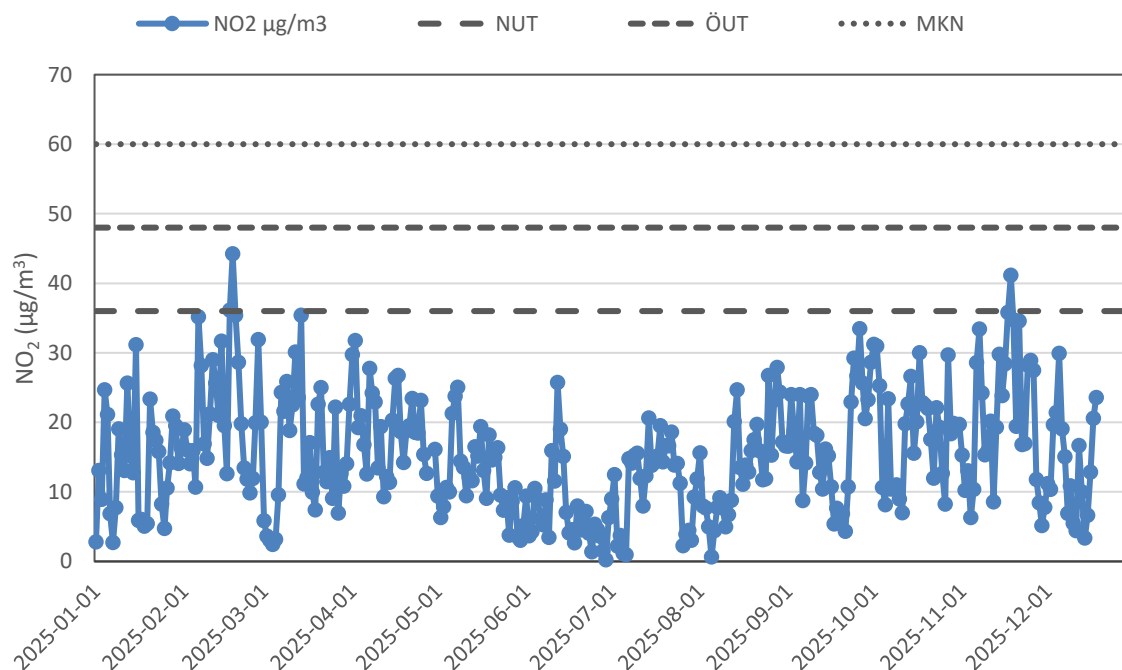
Figur 10 Dgnsmedelvärden av kvävedioxidhalter i µg/m 3 vid mätstationen Borås Kungsgatan under år 2025.
