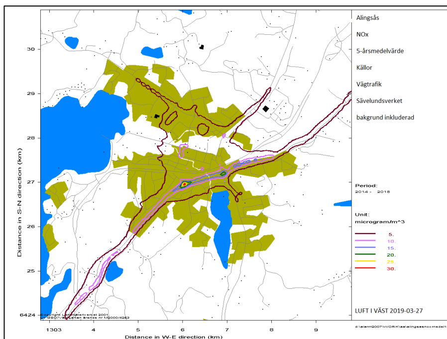
Figur 1 Resultat av en spridningsberäkning av årsmedelvärden kväveoxider (kväveoxid + kvävedioxid) i Alingsås tätort baserat på data från perioden 2014–2018. Modellsystem: ALARM.
