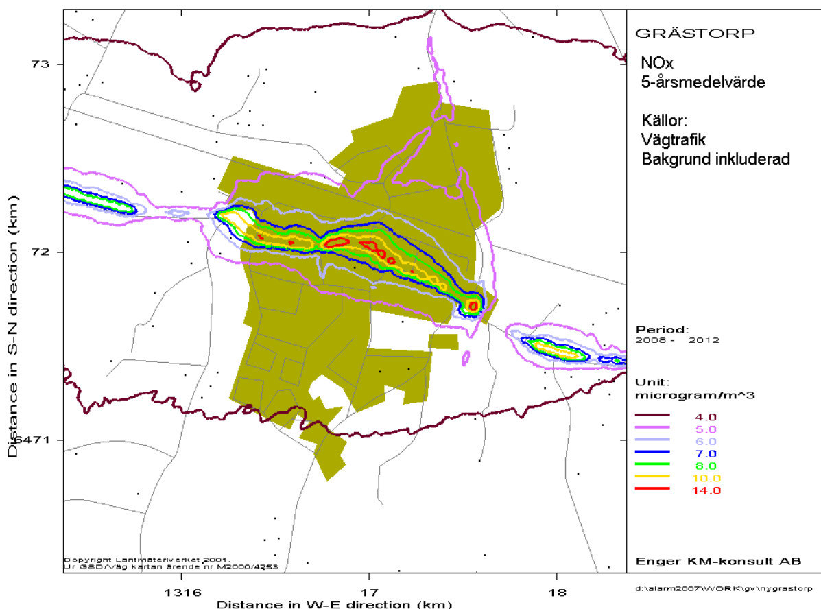
Figur 1 Resultat av en spridningsberäkning av femårsmedelvärde för kväveoxider (kväveoxid + kvävedioxid) i tätorten Grästorp baserat på data från perioden 2008–2012. Modellsystem: ALARM.
