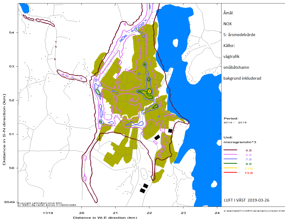
Figur 1 Resultat av en spridningsberäkning av årsmedelvärde för kväveoxider (kväveoxid + kvävedioxid) i tätorten Åmål baserat på data från perioden 2014–2018. Modellsystem: ALARM.
